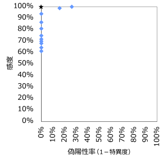
【ROC解析】
