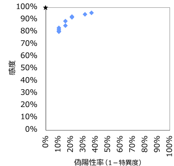
【ROC解析】
