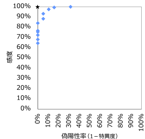
【ROC解析】
