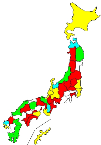
530 例 Coxsackievirus A6
