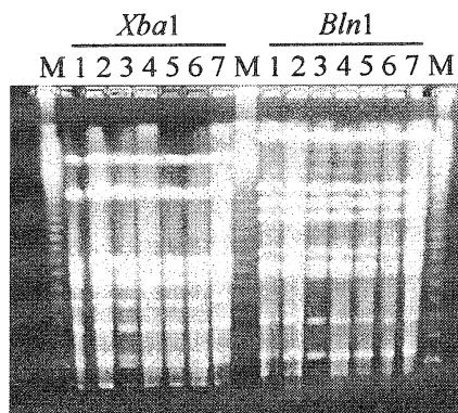
図 S. Enteritidis 分離株の PFGE パターン
