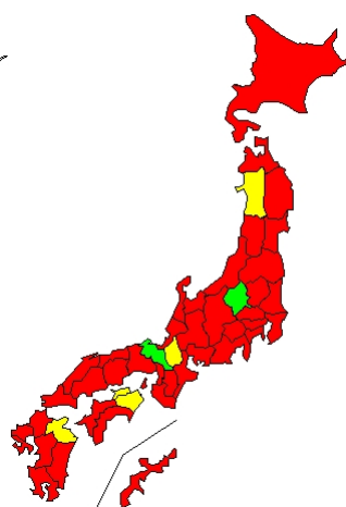
1716 cases A(H3)
