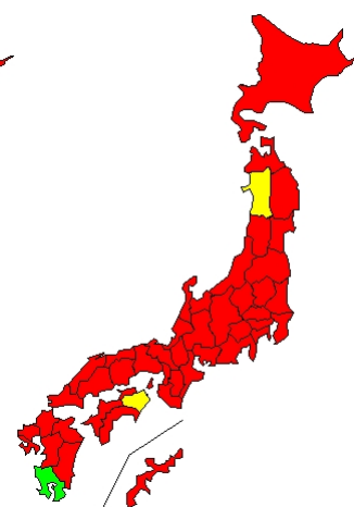
2949 cases B(Total)
