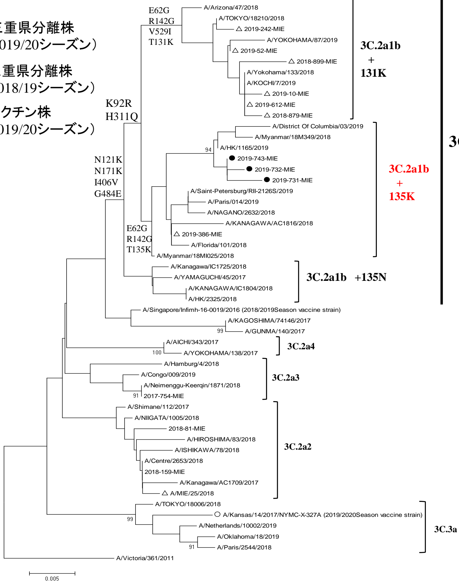
図2 AH3亜型インフルエンザウイルス HA遺伝子系統樹解析
